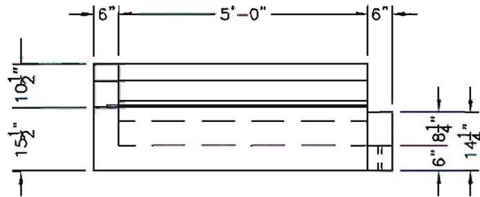
ELEVATION A-A
