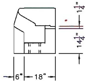
ELEVATION B-B
